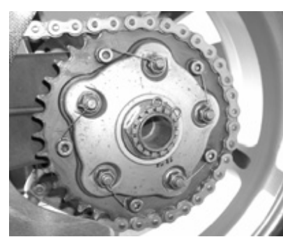
ワイヤーロック例：スプロケットナット
