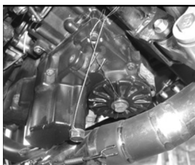
ワイヤーロック例：オールドレンボルト
