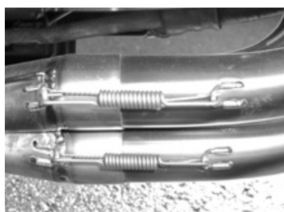
ワイヤーロック例：マフラージョイント (ワイヤーは、スプリングの中心部を通す。)
